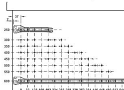
Padrão de furação
